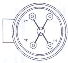
Рисунок 3. Нумерация клемм контактной колодки термообразователя.
